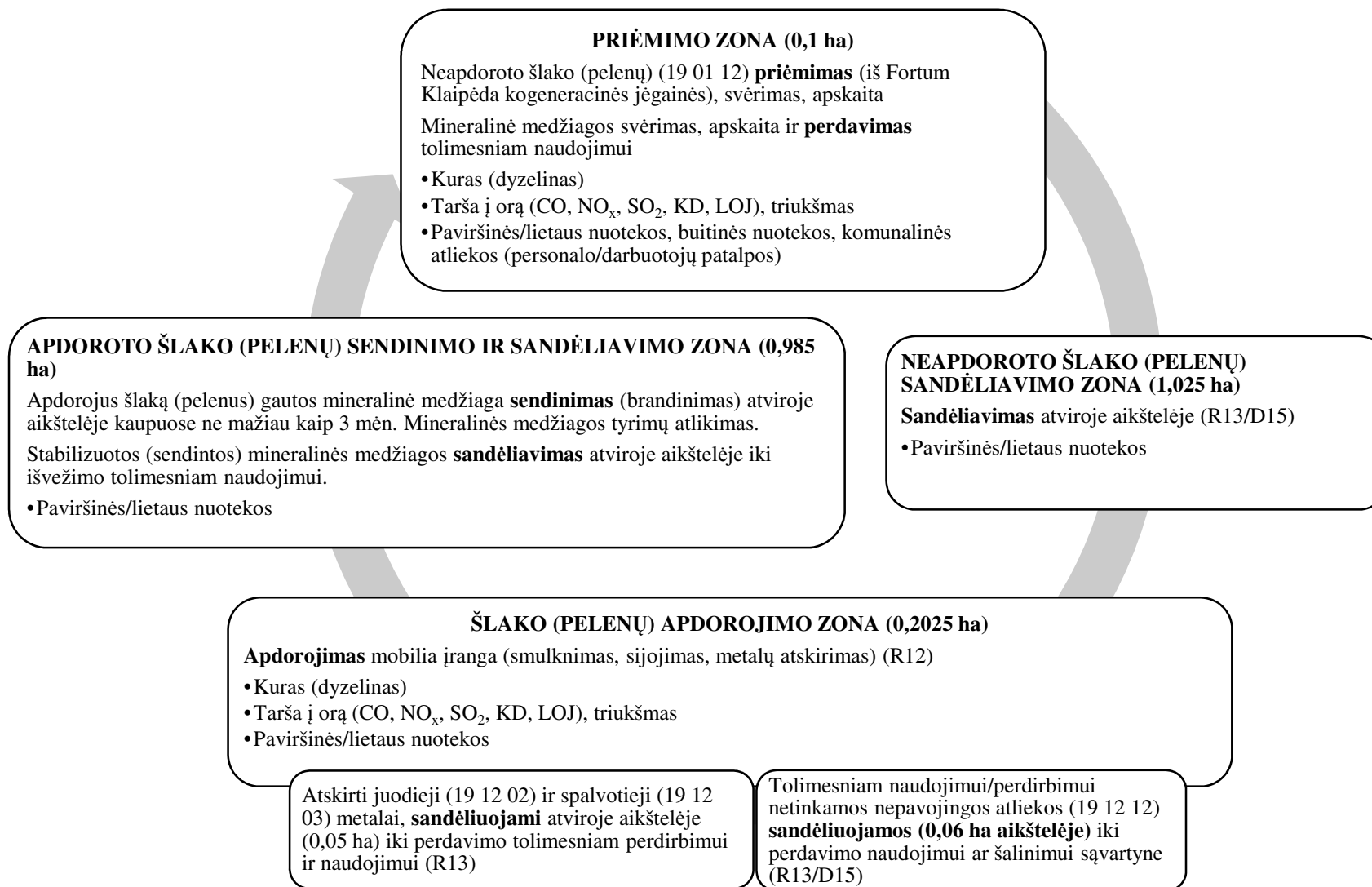
3 pav. Šlako (pelenų) apdorojimo aikštelėje PŪV principinė technologinė schema
